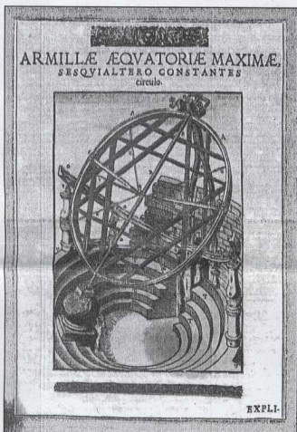
Tycho de Brahe: Astronomiae instauratae mechanica (1598)
