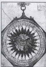
Petrus Appianus: Astronomicum Caesareum (1532)
